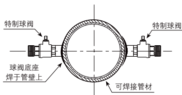
焊接固定球阀底座
