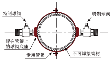
管箍固定球阀底座
