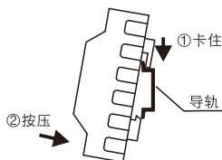
安装图
